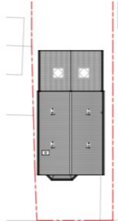
③ Roof Plan 1 : 100
